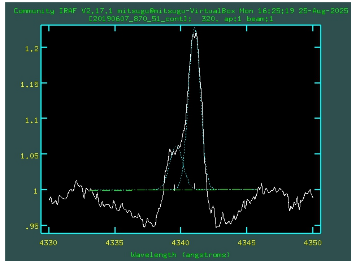
図4 観測スペクトル(白)に対してガウスフィットで2成分に分離(緑破線)。 左2019/6/7 右2025/3/19 こういう方法で良いかどうか？ また完全にシングルピークの日があったが、その日のV/Rは1とした。
