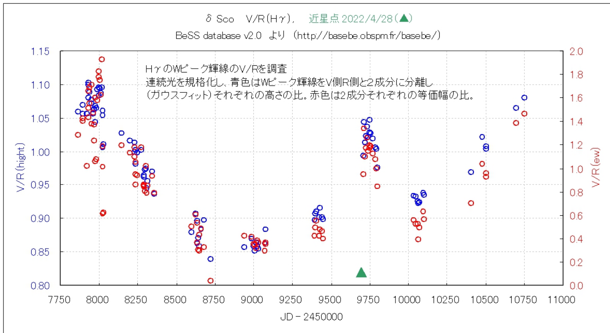
図1 V/R比 青色はガウスフィット後の高さ測定、赤色はガウスフィット後の等価幅測定。 ▲印は伴星の近星点通過日で、2017/4/20-2025/3/19までの約8年間の98夜分を示す。
