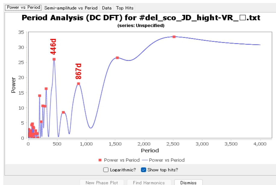
図2 高さを測定したV/Rの周期解析
