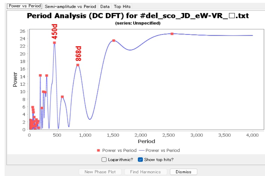
図3 等価幅を測定したV/Rの周期解析
